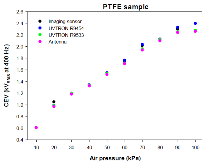
1-сурет. 10-100 кПа қысым диапазонында әртүрлі датчиктермен ПТФЭ оқшаулауы бар сым электродтарында анықталған тәждік разрядтың өшу кернеуінің мәндері (CEV)
